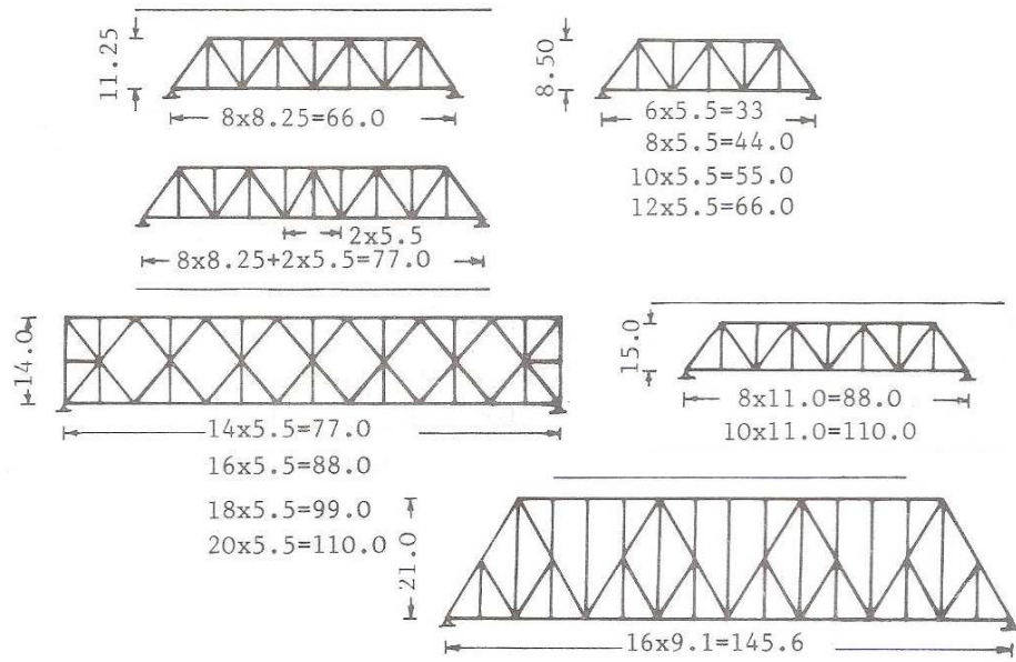
أشكال الجوائز الشبكية النموذجية المستخدمة في جسر طرق السيارات
